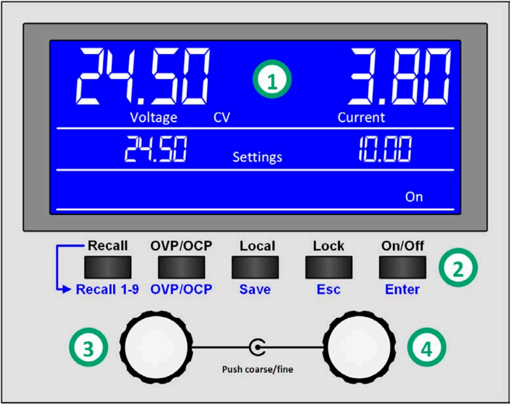
图 5 - 控制面板
