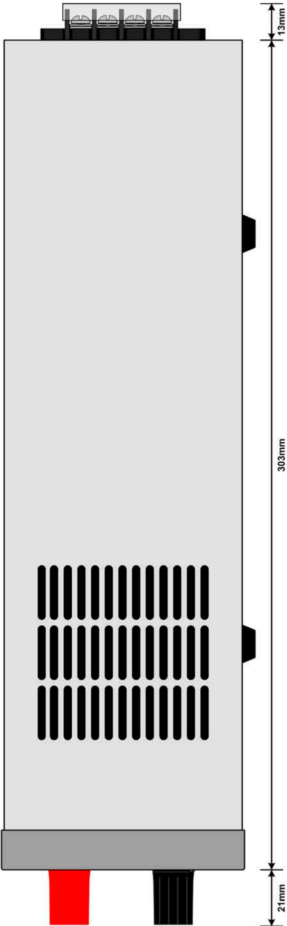
图 4 - 160W/320W型号右侧视图
