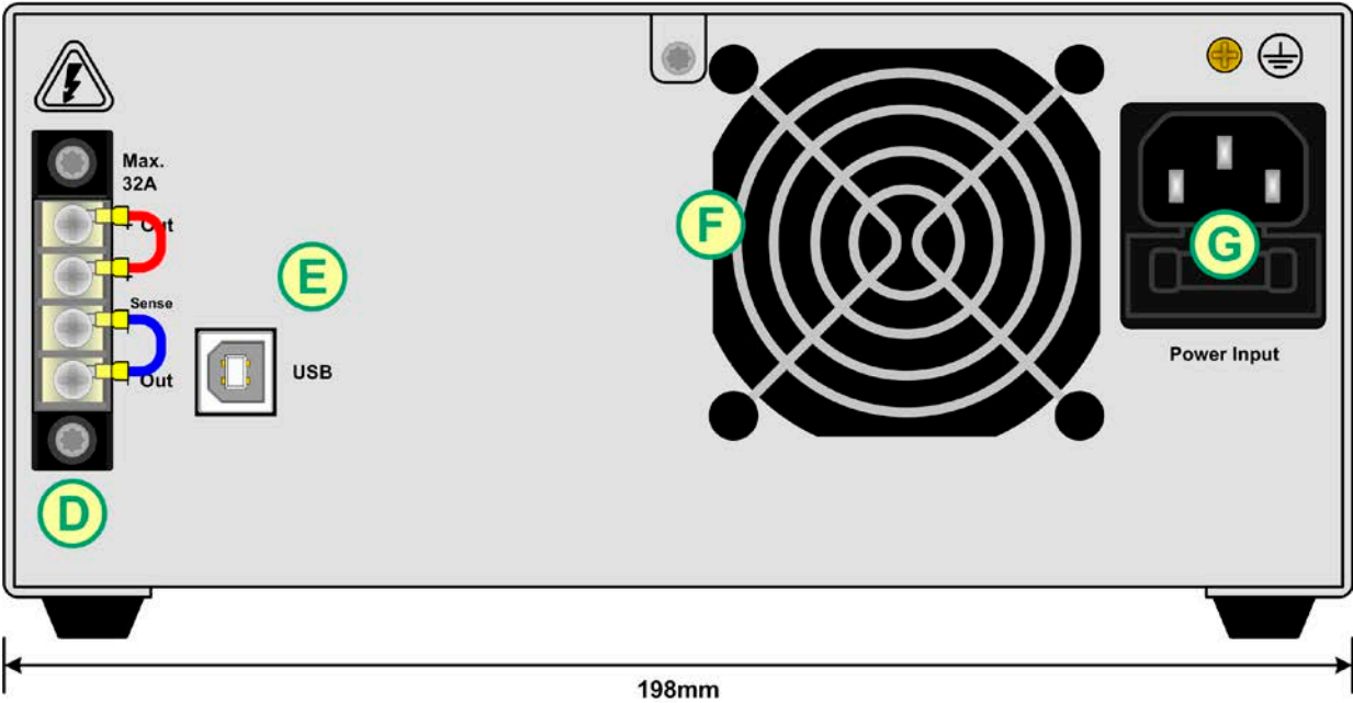
图 2 - 后视图
