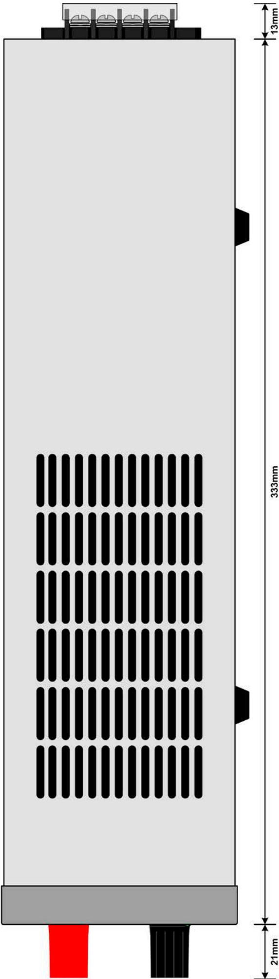
图 3 - 640W型号右侧视图
